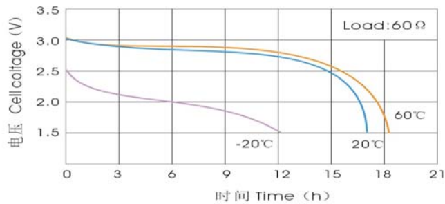
常温负载特性 Discharge Characteristics
