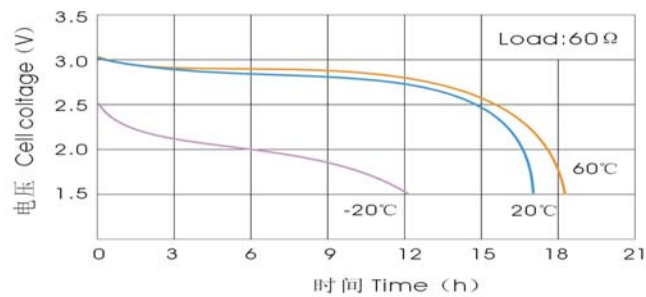
常温负载特性 Discharge Characteristics
