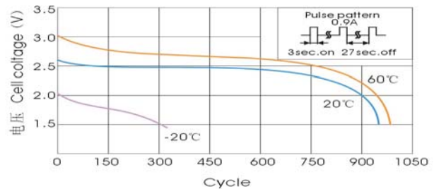
脉冲放电特性 Pulse Discharge Characteristics
