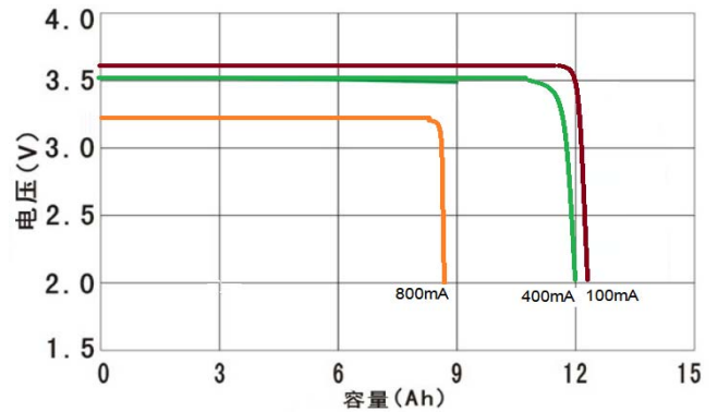
1. 在+135°C下典型放电曲线 (中间值)
